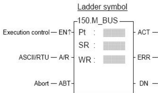
Rys. 8 Symbol funkcji 150.M_BUS
