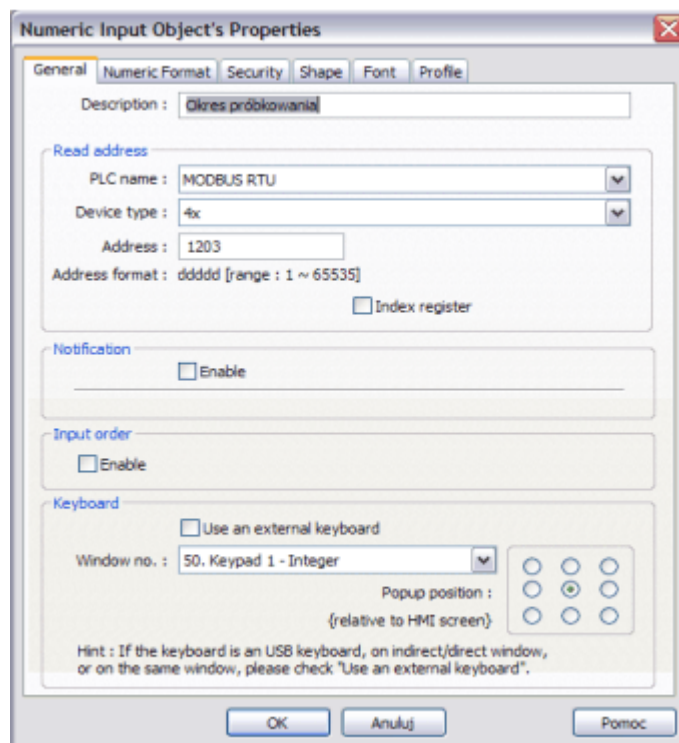
Rys. 19 Właściwości obiektu Numeric Display
