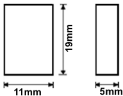
Rys. 22 Wymiary czujnika MCTH-2
