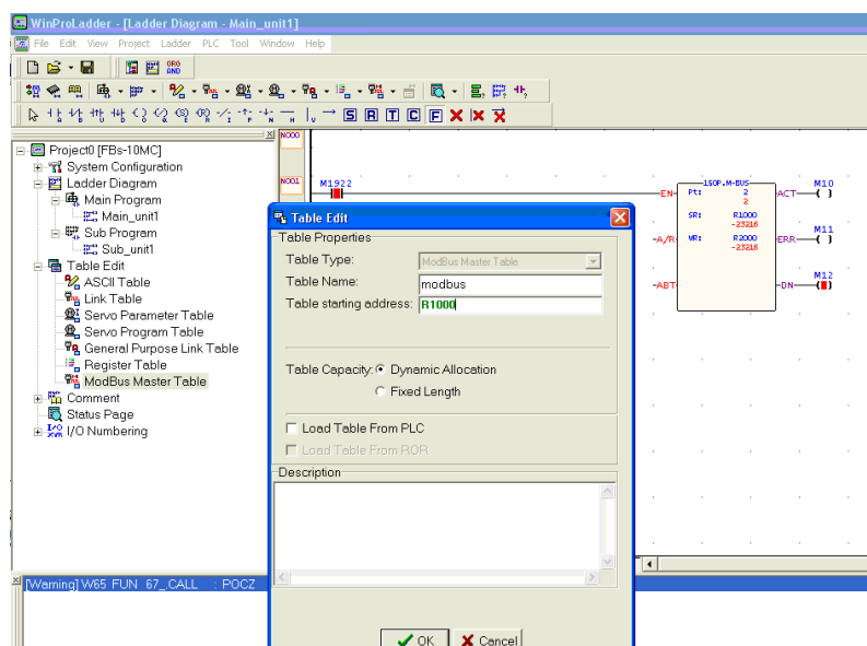
Rys. 11. Okno konfiguracji funkcji Modbus w sterowniku FATEK.
