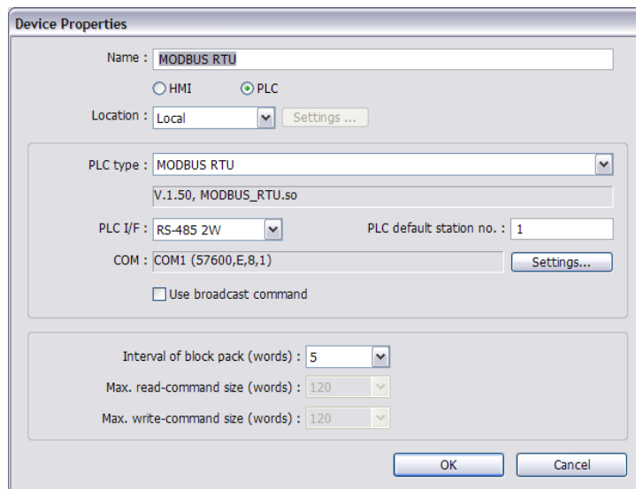
Rys.14 Okno do edycji parametrów komunikacji
