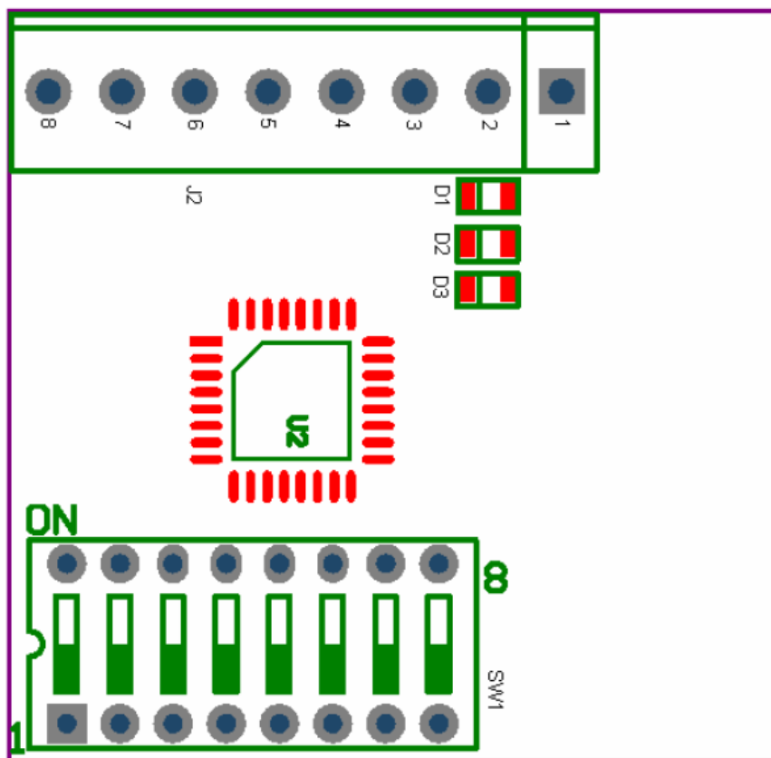
Rys. 2. Rozmieszczenie elementów na płytce modułu
