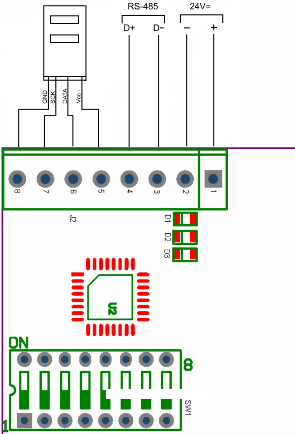
Rys. 3 Przykład połączenia modułu MCTH-1
