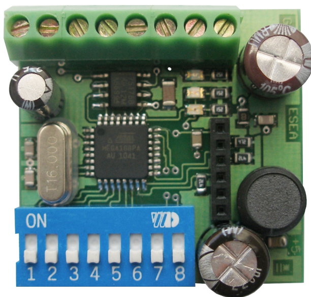
Rys. 1. Widok modułu MCTH-1
