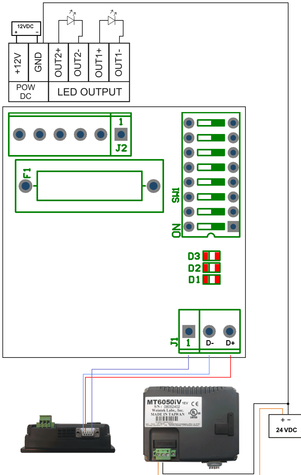
Rys. 17. Schemat podłączenia ściemniacza LED SCL-2P do panelu HMI firmy Weintek
