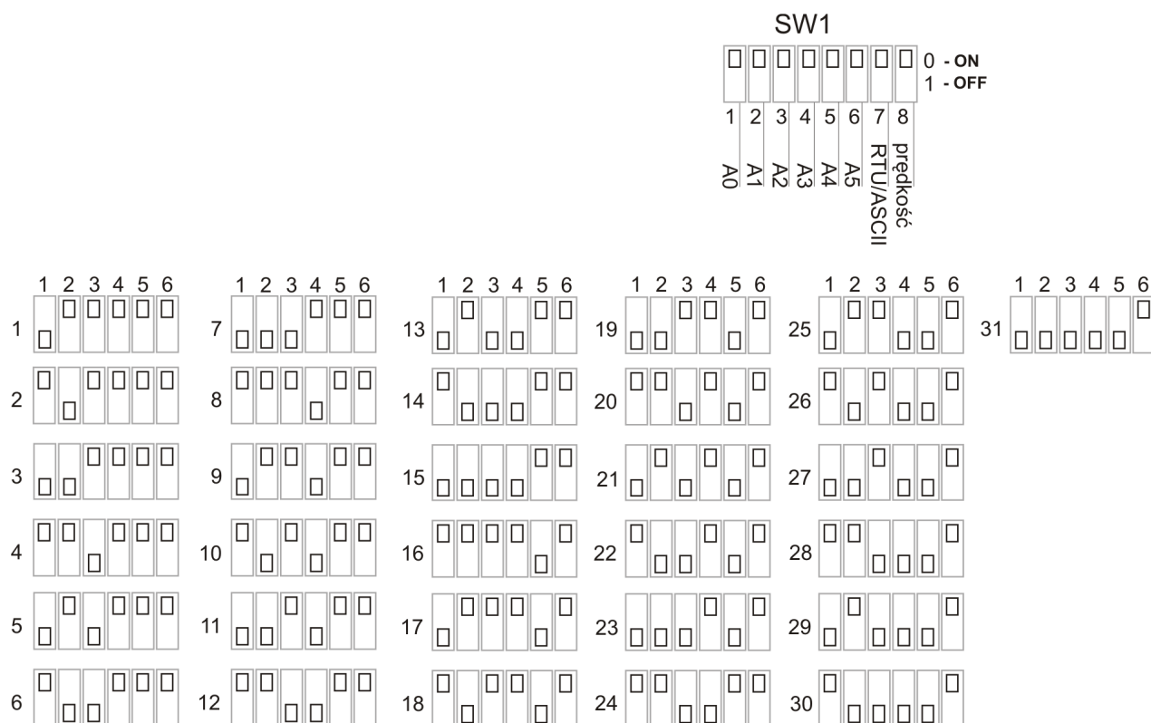
Rys. 8 Zworki SW1 do ustawiania adresu Modbus (zworki 1-6). Na rysunku przedstawiono 31 z 63 możliwych ustawień adresu.
