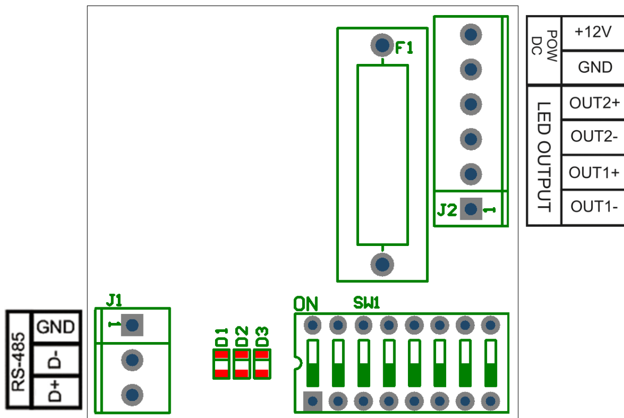
Rys. 2. Rozmieszczenie konektorów ściemniacza LED SCL-2P. Widok płytki.
