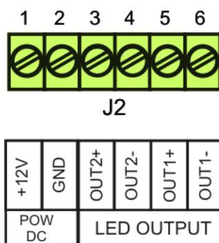
Rys. 4. Widok złącza zasilającego - wyjściowego J2 ściemniacza LED SCL-2P.
