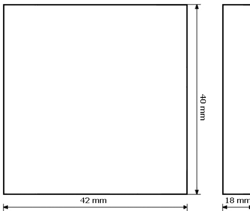
Rys. 6. Wymiary ściemniacza LED SCL-2P
