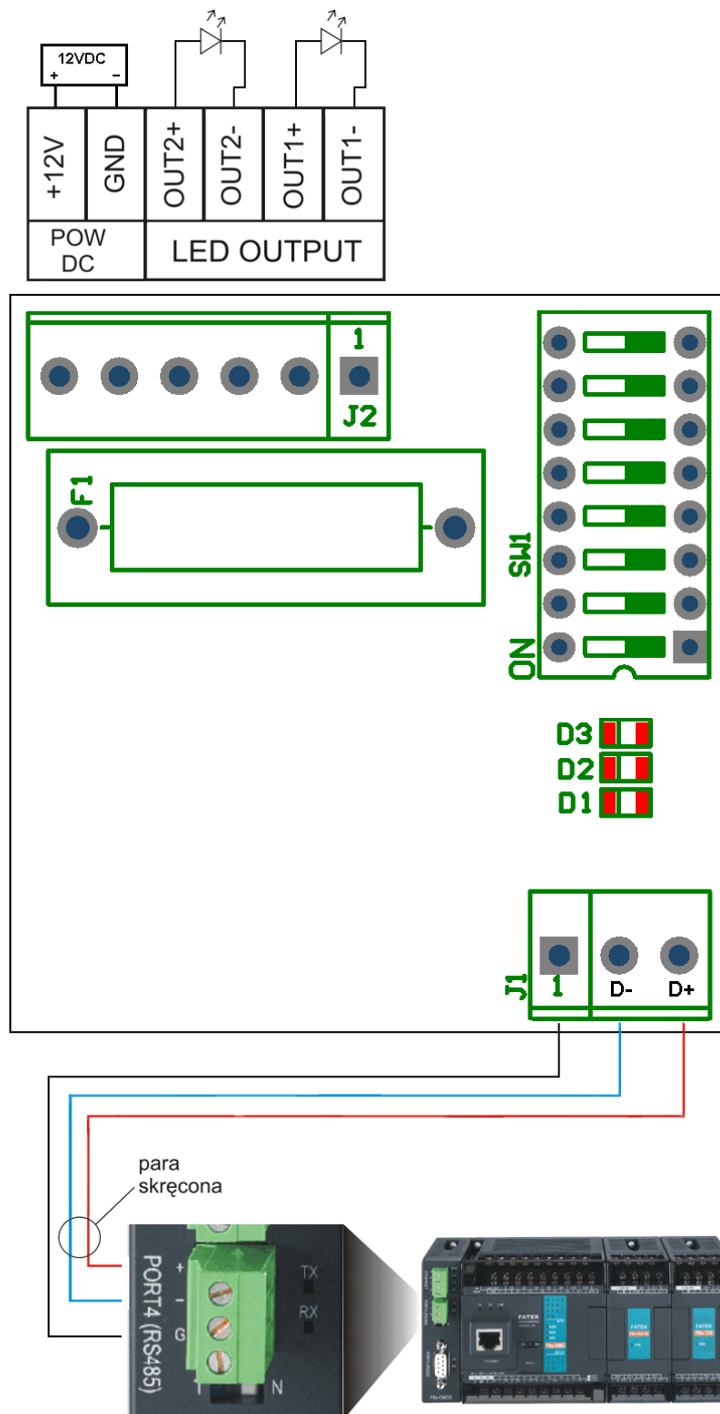
Rys. 5. Przykład typowego podłączenia ściemniacza LED SCL-2P do sterownika PLC
